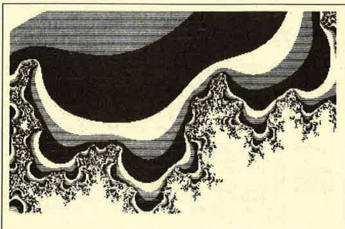
Beispiel Mandelbrotmenge, Zeit 3:43 min
